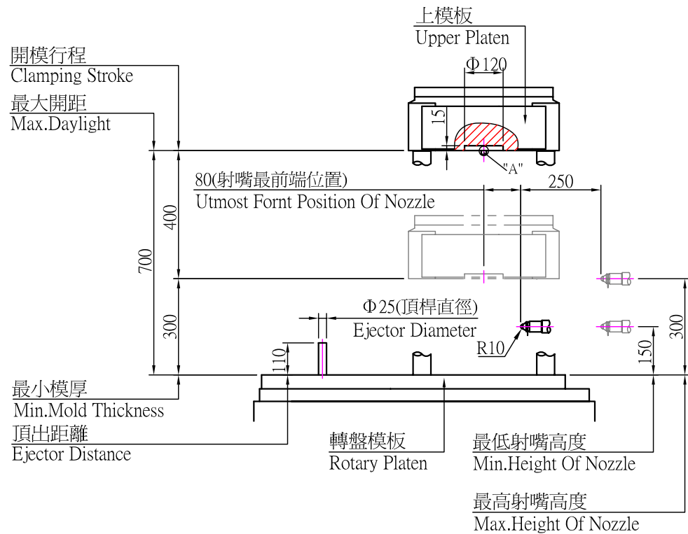
開合模規格示意圖(Clamping Unit Diagram)
