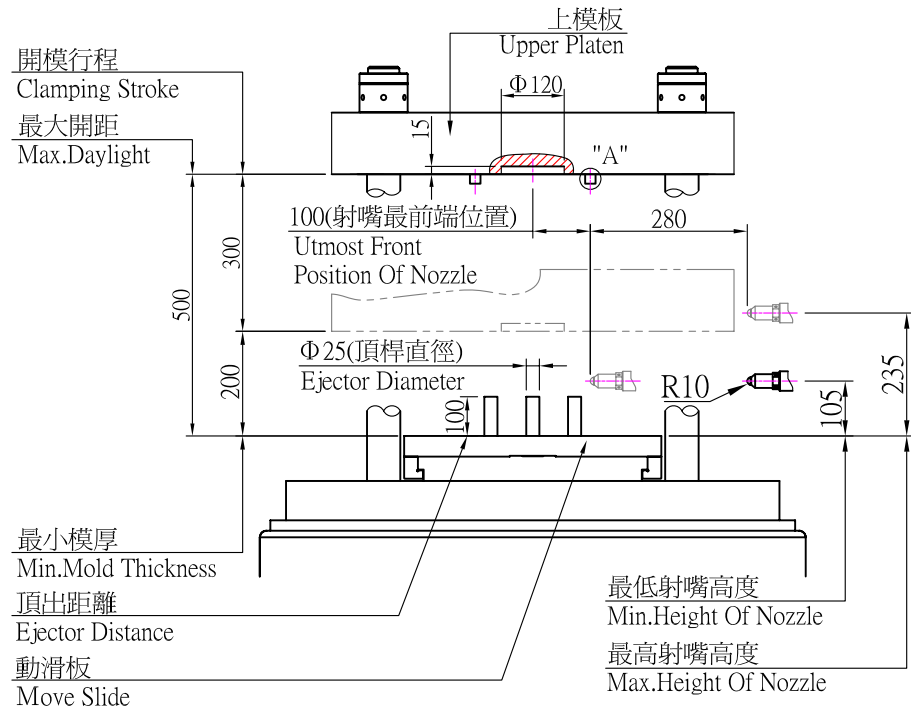
開合模規格示意圖(Clamping Unit Diagram)
