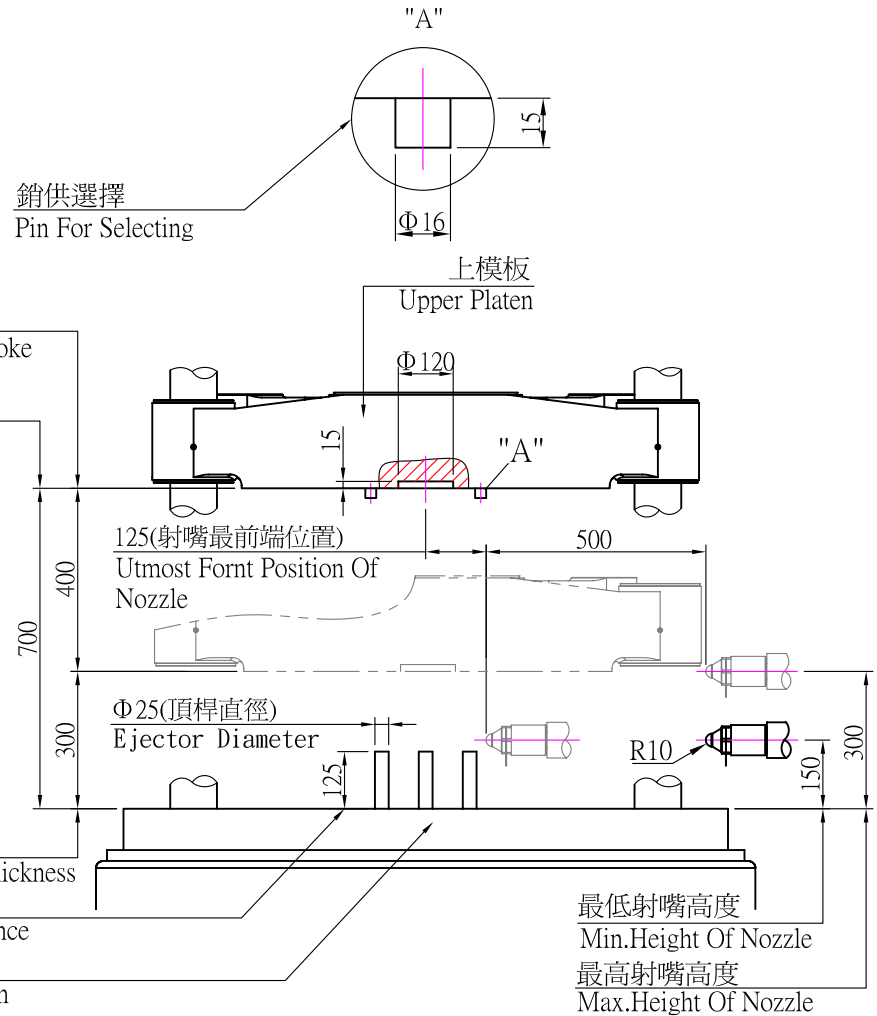
開合模規格示意圖(Clamping Unit Diagram)
